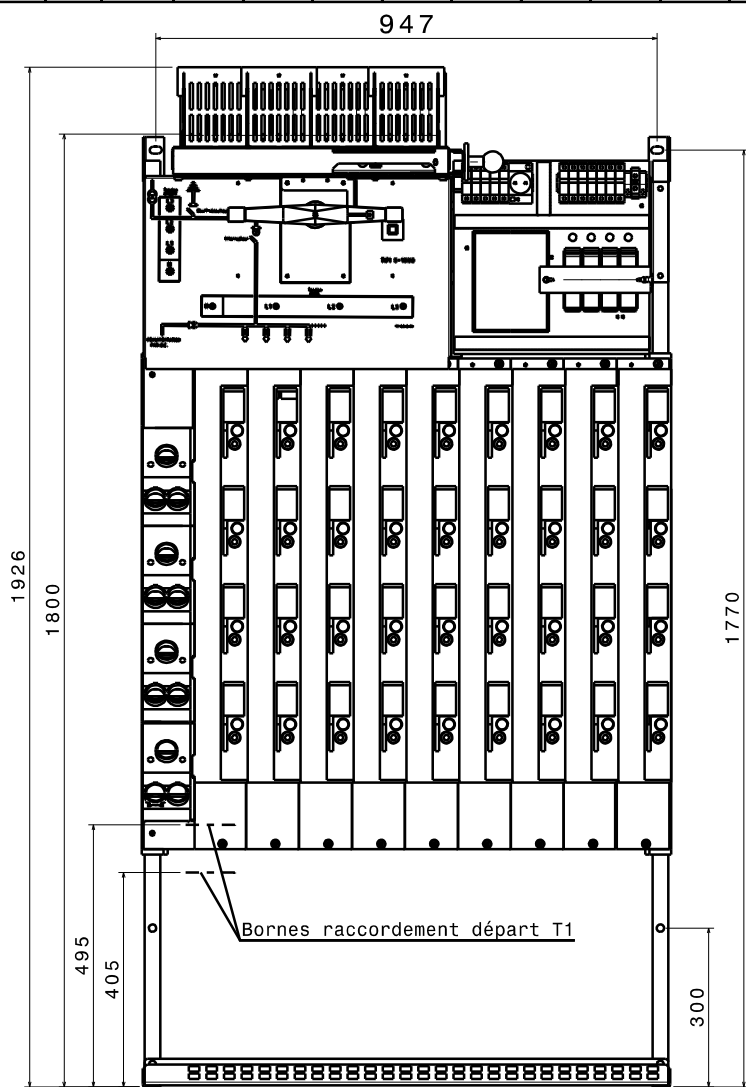
Vue de face Echelle : 1:5
