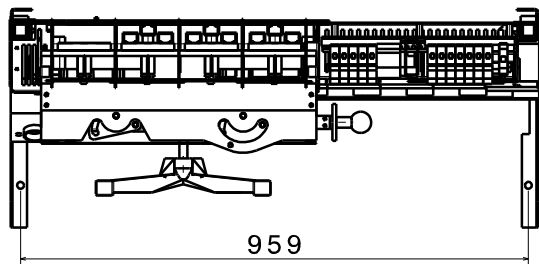
Vue de dessus Echelle : 1:5
