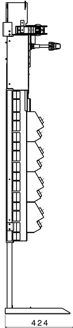
Vue de gauche Echelle : 1:5
