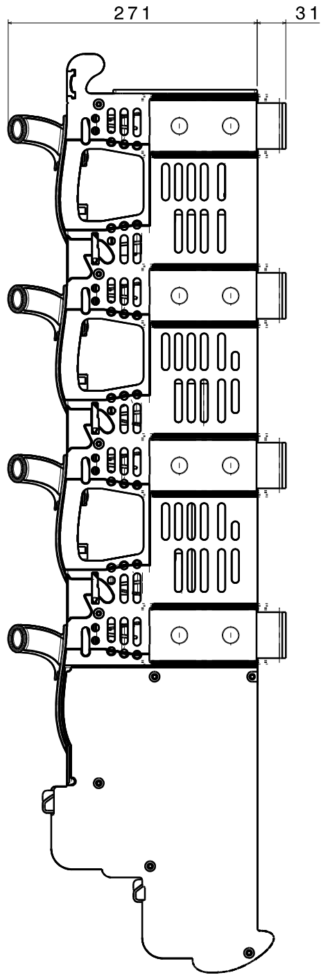
Vue de face Echelle : 1:2
