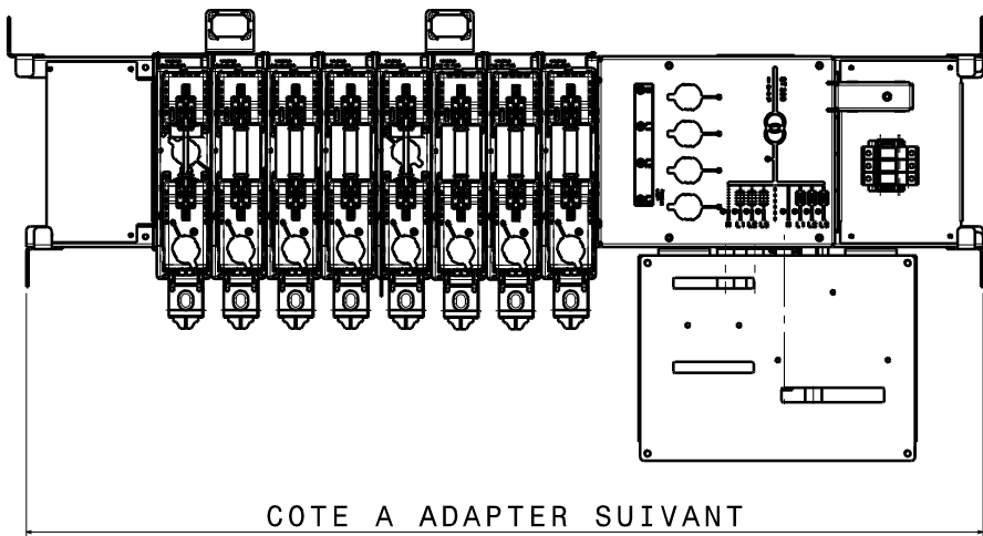
Vue de face Echelle : 1:4
