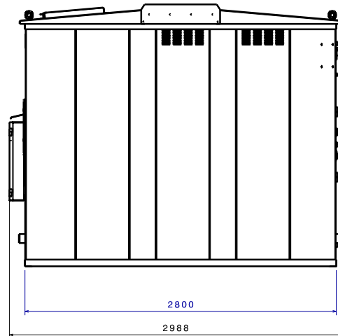
Vue de gauche Echelle : 3:50
