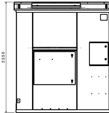
Vue arrière Echelle : 3:50
