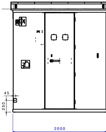
Vue de face Echelle : 3:50
