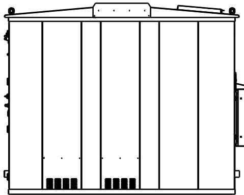
Vue de droite Echelle : 3:50
